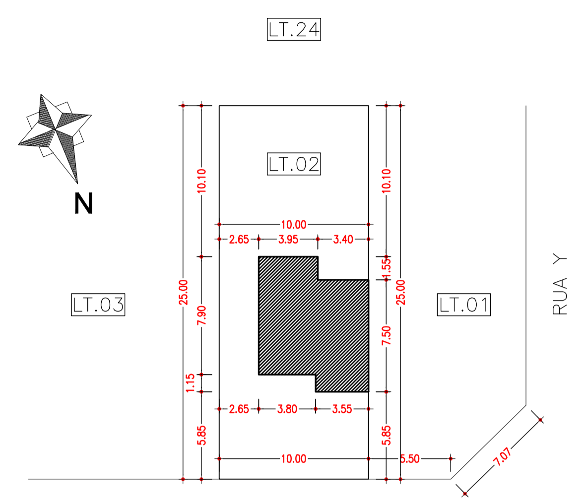
LOCAÇÃO/SITUAÇÃO ESC.: 1:250
