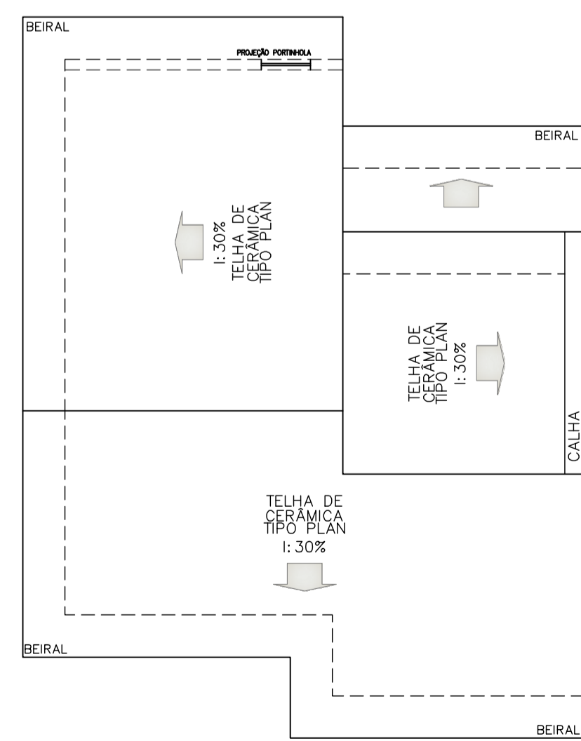
COBERTURA ESC.: 1:100
